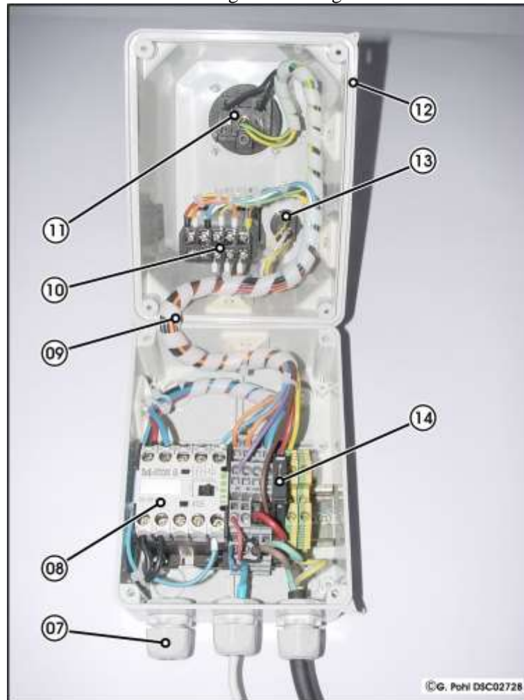
Verdrahtungsansicht Regler RT1
