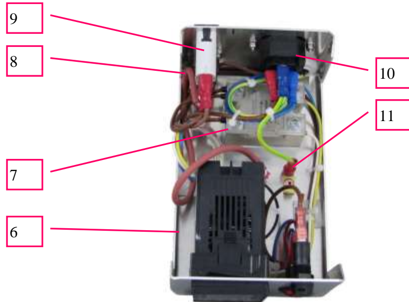
Gesamtansicht Regler RT5-19
