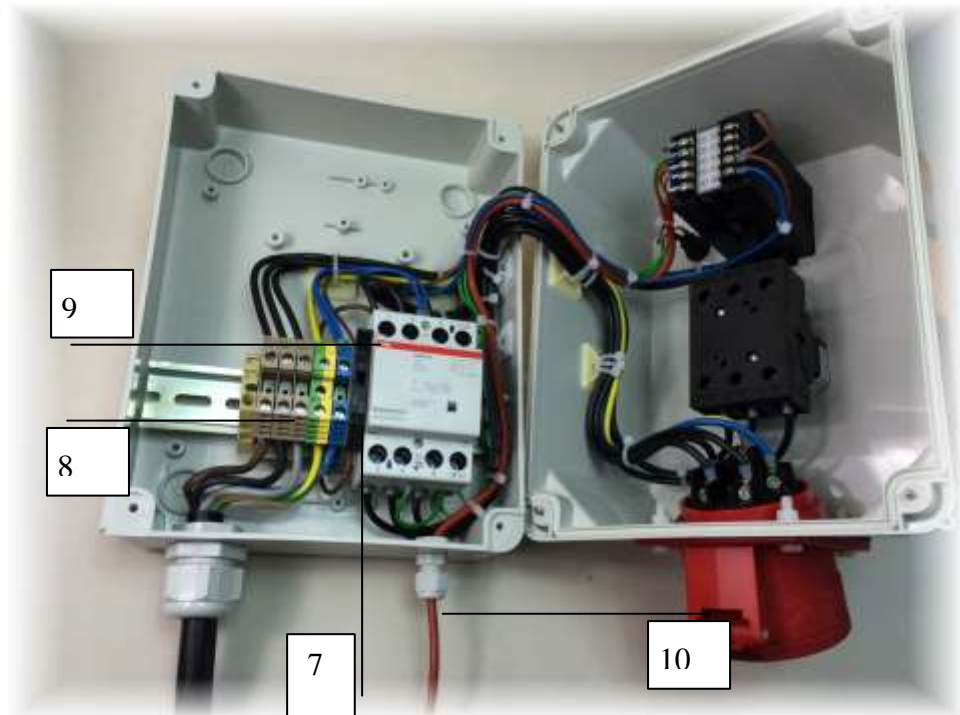
Verdrahtungsansicht Regler RT2-56-(beispielhaft)
