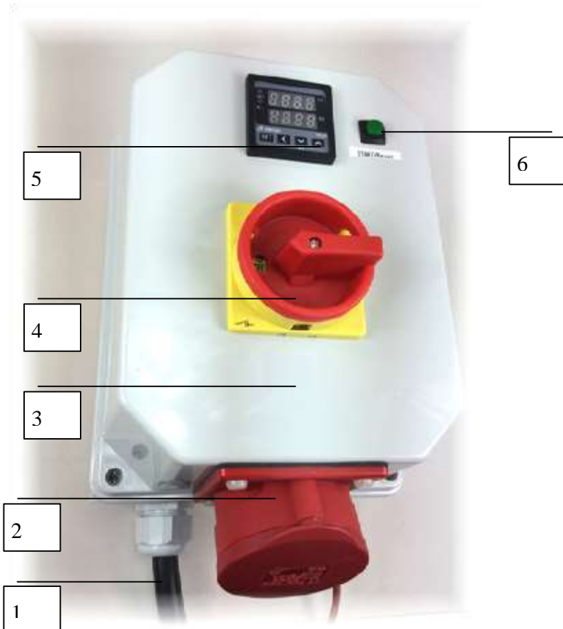
Gesamtansicht Regler RT2-56 – (Beispielhafte Abb)
